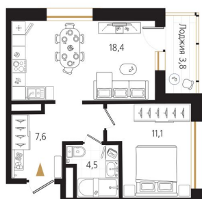
КОРПУС А2 14 этаж
