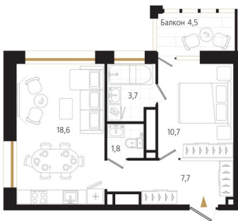
КОРПУС С1 20 этаж
