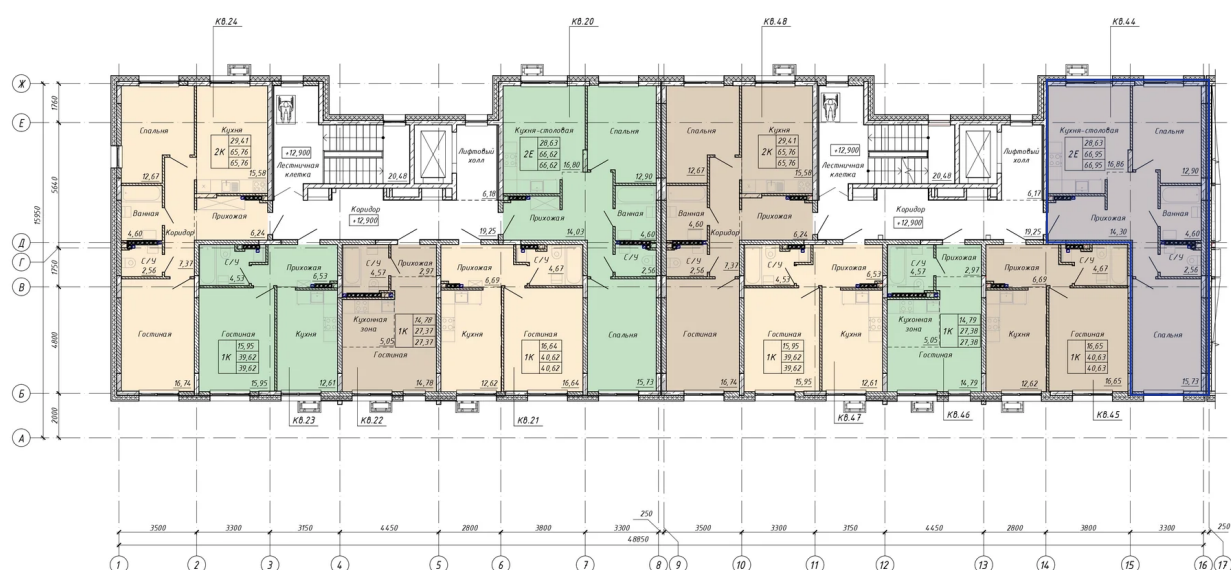
Поэтажные планы 5 этажа дома №1 (ОКС-1.1) Секция 1,2 Подъезд 1,2
