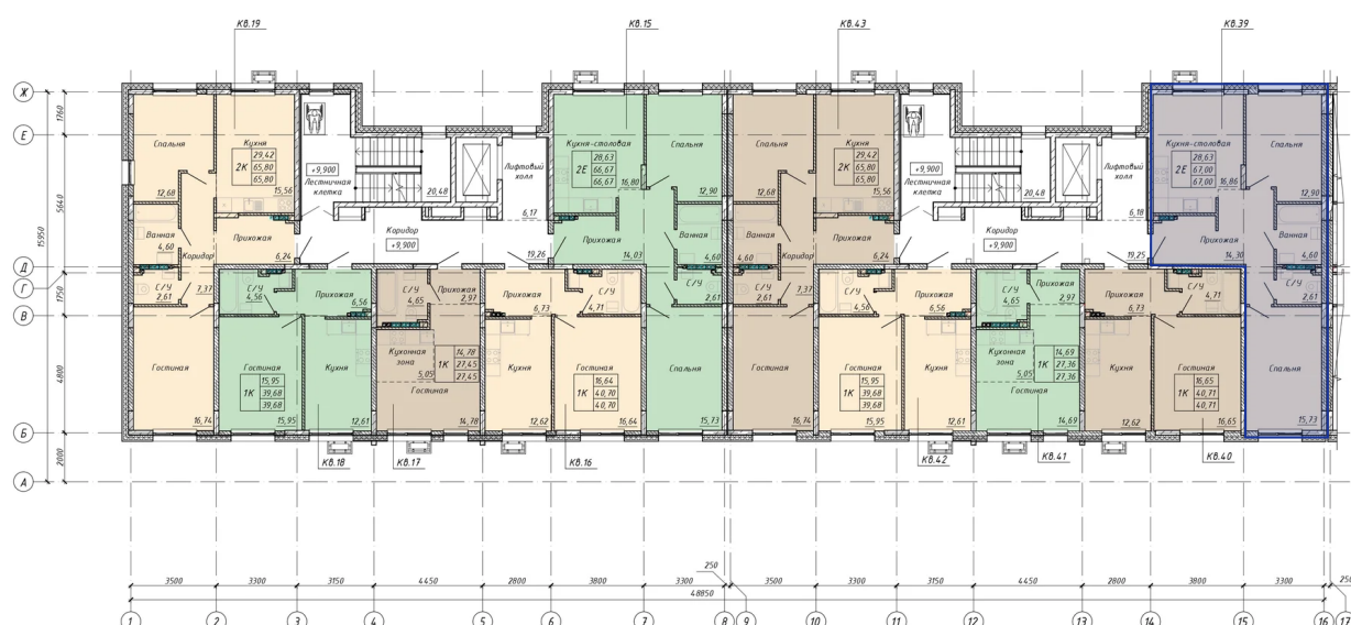
Полэтажные планы 4 этажа дома №1 (ОКС-1.1) Секция 1,2 Подъезд 1,2
