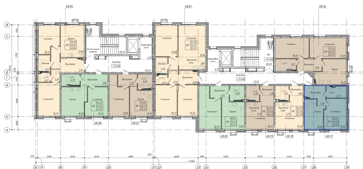
Поэтажные планы 4 этажа дома №1 (ОКС-1.1) Секция 3,4 Подъезд 3,4
