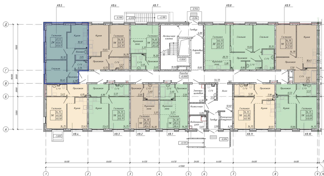
Поэтажные планы 1 этажа дома №3 (ОКС-1.3) Секция 1 Подъезд 1
